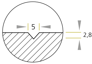
Pico de Gorrión Birdsmouth joint Bec de moineau
