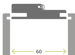
Batientes / Tapetas extensibles Adjustable frame / Architraves Chambranles / Couvre-joints coulissants
