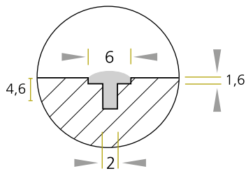
Inserción en aluminio Aluminium inlay Insertion en aluminium
