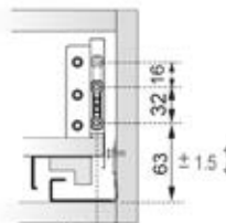
Montaje frontal
