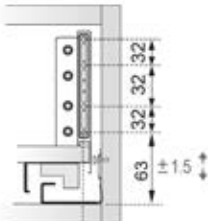
Montaje frontal
