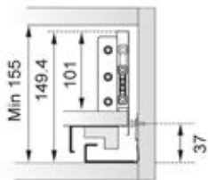
Montaje Mínimo
