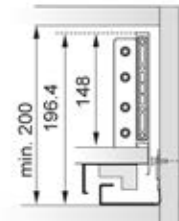
Montaje Mínimo
